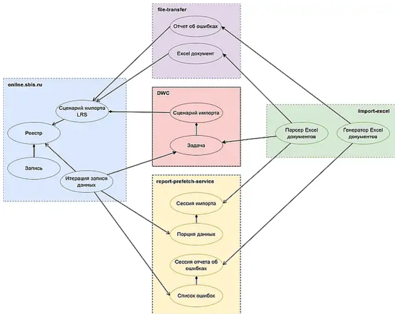
Схема 1. Взаимодействие сервисов
